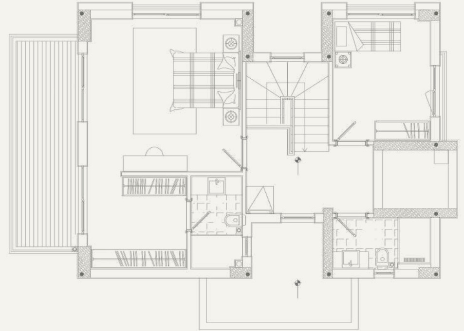
02 / 1. KAT
